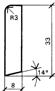
Smyglist 33
