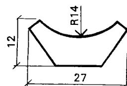
Hålkäl 27
