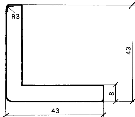
Hörnlist 43
