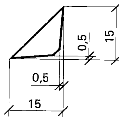
Trekantlist 15
