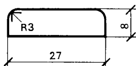
Foglist 8x27
