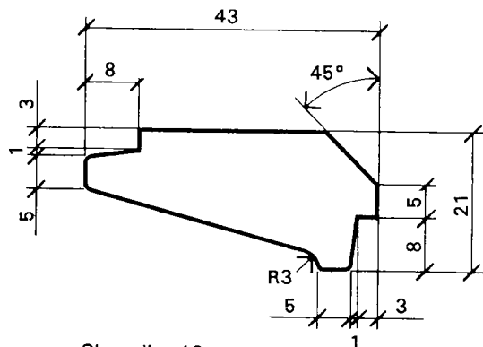
Skugglist 43
