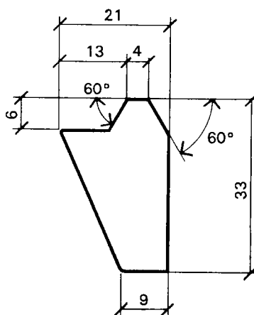
Skugglist 21
