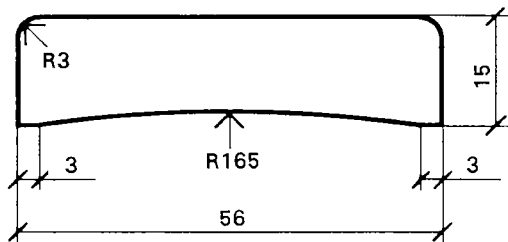
Foderlist 15x56
