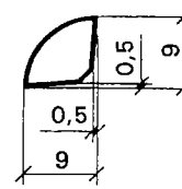
Kvartlist 9
