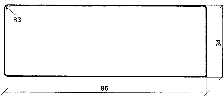
Trälläkt 34x95
