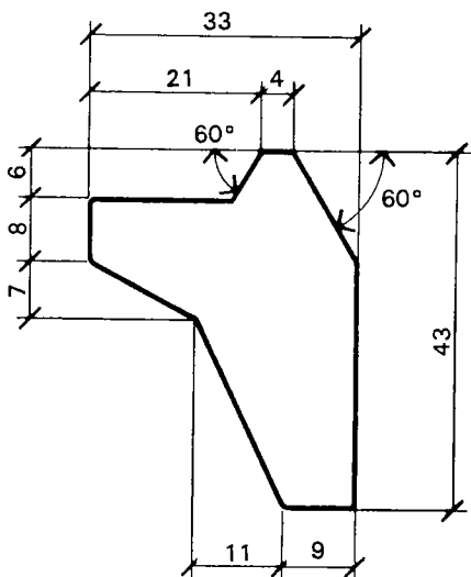
Skugglist 33
