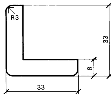
Hörnlist 33
