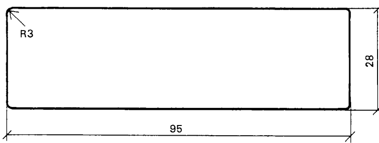
Trälläkt 28x95
