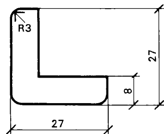
Hörnlist 27
