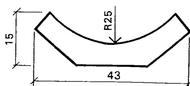
Hålkäl 43
