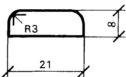
Foglist 8x21
