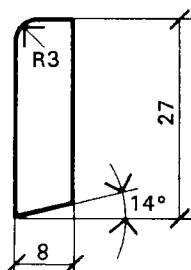
Smyglist 27
