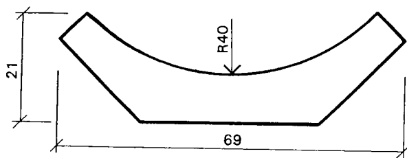
Hålkäl 69
