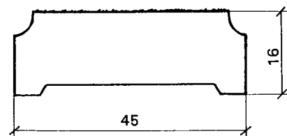
Allmogelockläkt 16x45
