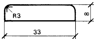
Foglist 8x33
