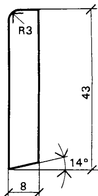
Smyglist 43
