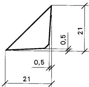
Trekantlist 21
