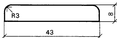
Foglist 8x43
