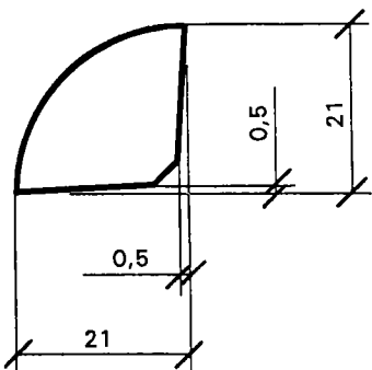
Kvartlist 21
