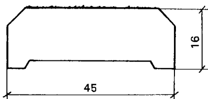
Lockläkt 16x45
