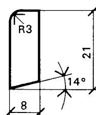
Smyglist 21
