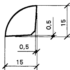
Kvartlist 15
