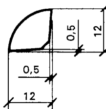
Kvartlist 12
