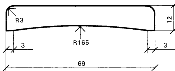
Foderlist 12x69
