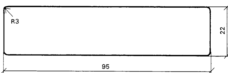
Trälläkt 22x95
