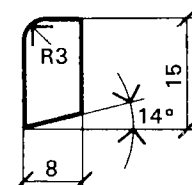
Smyglist 15
