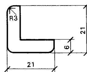
Hörnlist 21
