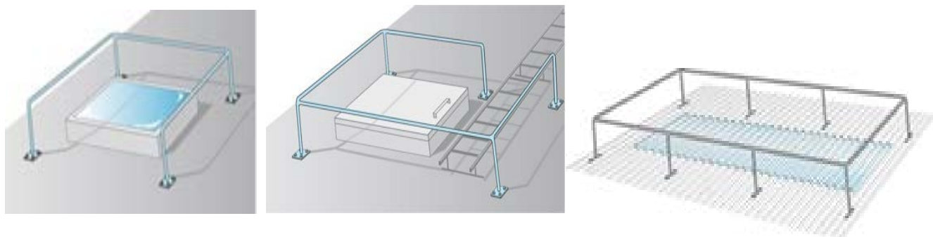
Figur 1– Exempel på utformning av räcken kring uppstigningslucka och takfönster
